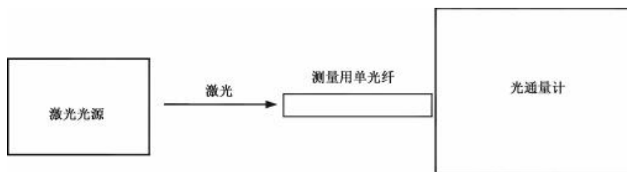
图 A.1 入射光的测量装置
