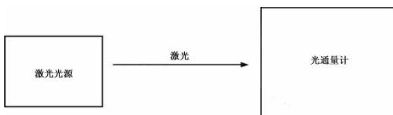
图 A.1 入射光的测量装置
