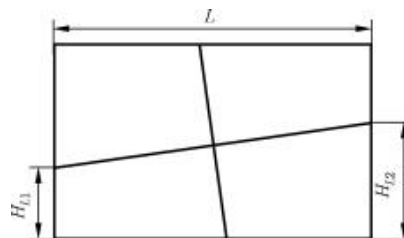
图 5 左右画面旋转边界相交示意图
