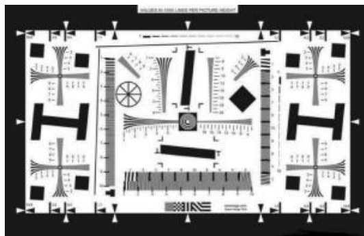
图 6 ISO 12233 分辨率测试图卡
